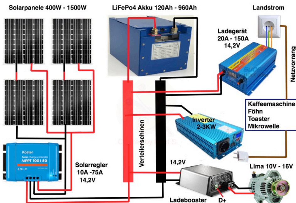
Anschluß-Übersicht (bei 24V Spannungswerte verdoppeln)
